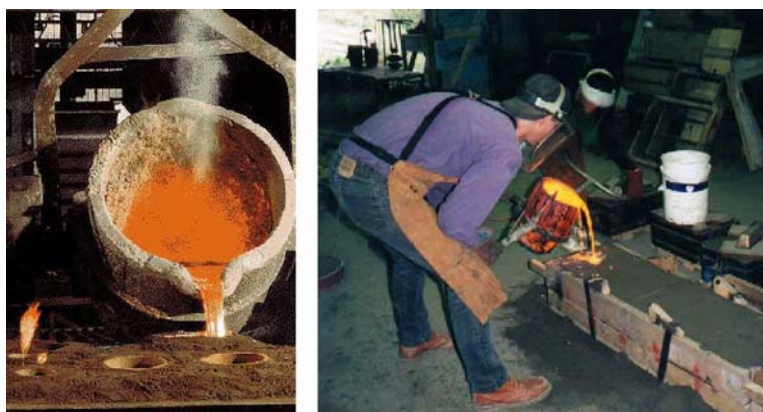
Σχήμα 1.4 : Χύτευση σε καλούπι από άμμο
