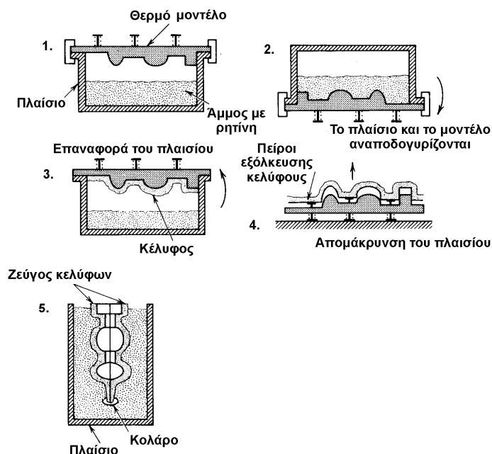
Σχήμα 1.5 : Χύτευση κελύφους
