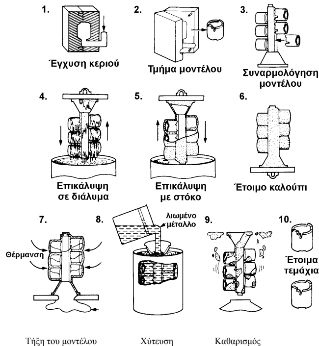
Σχήμα 1.6 : Χύτευση με την τεχνική του χαμένου κεριού.
