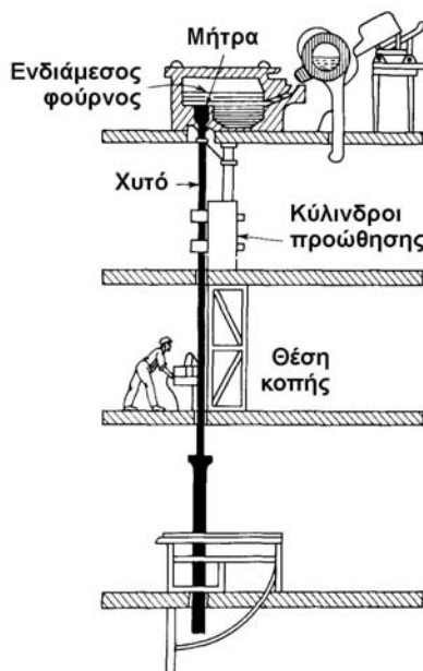
Σχήμα 1.9 : Συνεχής χύτευση
