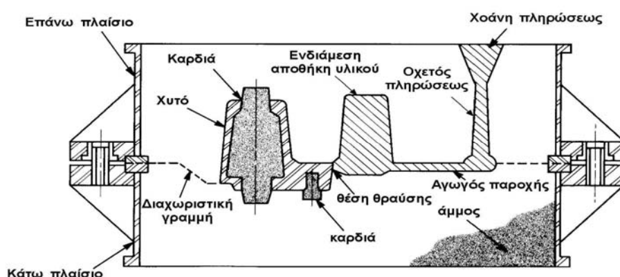
Σχήμα 1.2 : Καλούπι για χύτευση σε άμμο σε τομή
