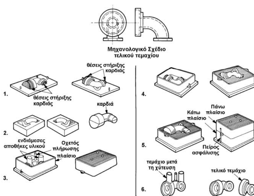
Σχήμα 1.3 : Χύτευση σε άμμο
