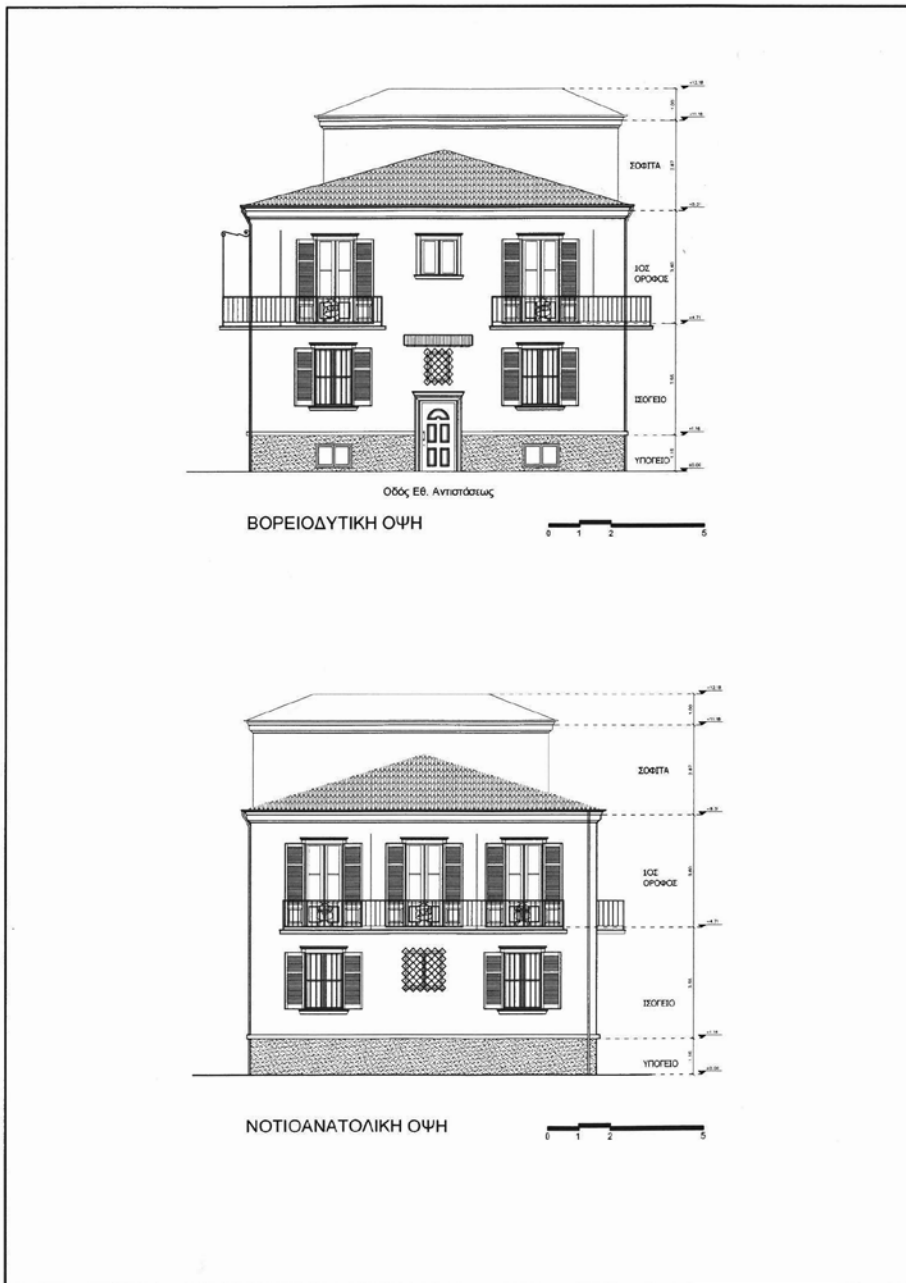
Εικ. 23: Βορειοδυτική και Νοτιοανατολική όψη (Σχέδιο Στ. Παπότη).
