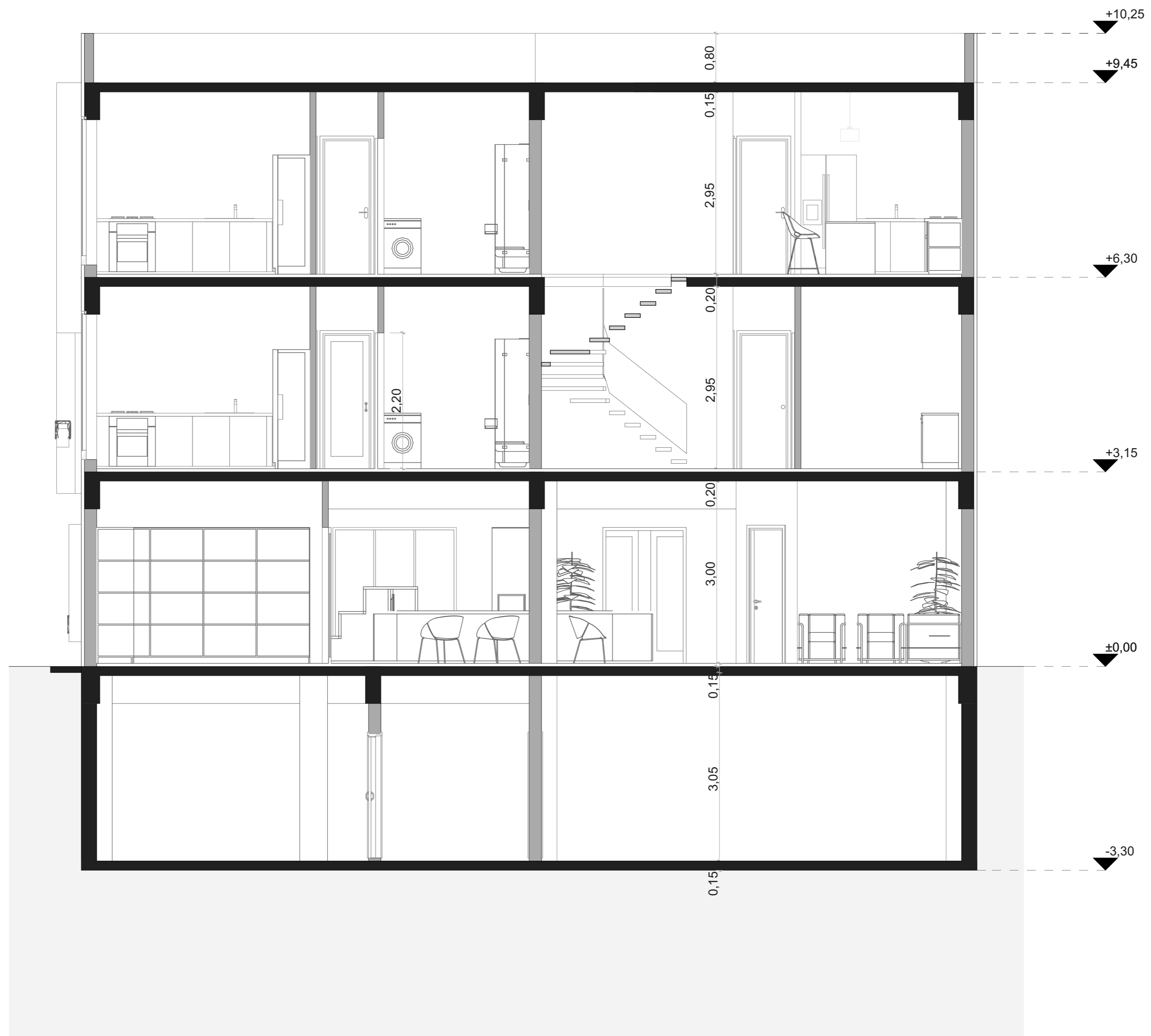
TOMH A1 ΚΑΙΜΑΚΑ 1:50
