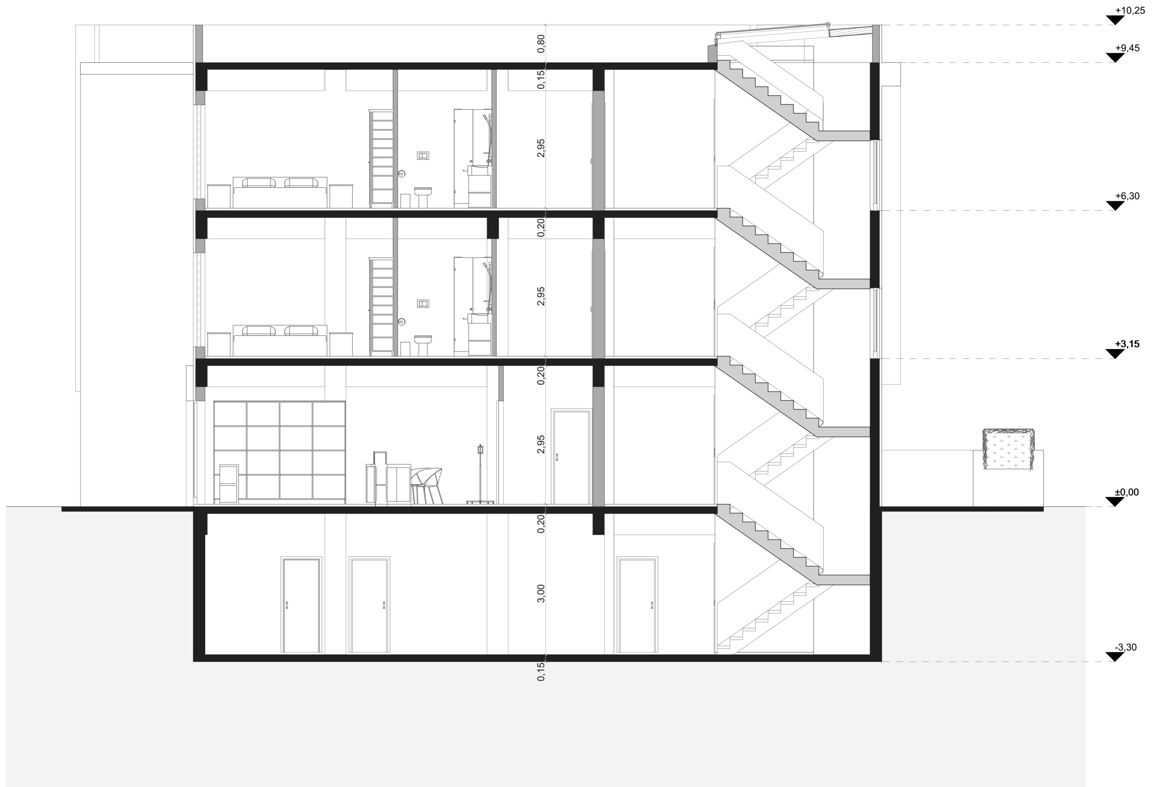
TOMH A2 ΚΛΙΜΑΚΑ 1:50
