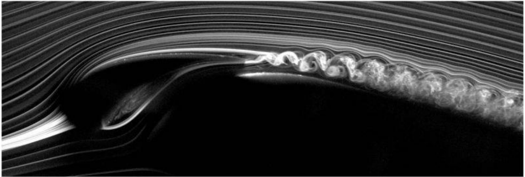
fig. 12 Δημιουργία δινών (vortex shedding trail) στο πίσω μέρος πτερυγίου.
