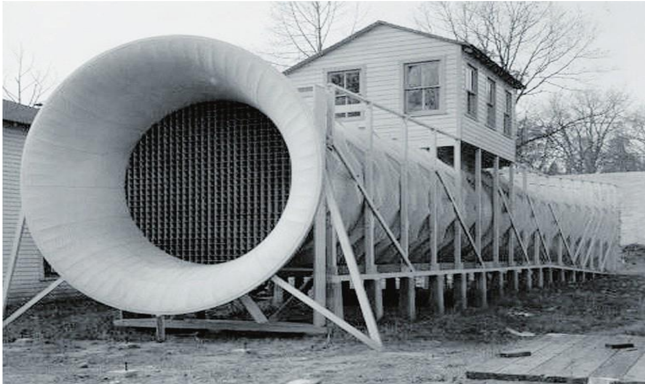
fig. 15 Πιστό μοντέλο της αεροσήραγγας του Francis Herbert Wenham.
