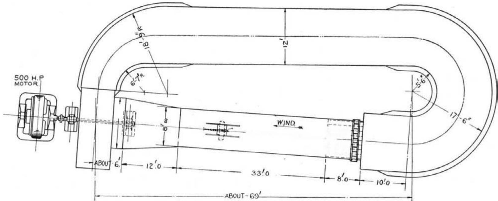
fig. 19 Διάγραμμα της αεροσφαιρα του πολεμικού ναυτικού Αμερικής. Washington, 8 Απριλίου 1916.
