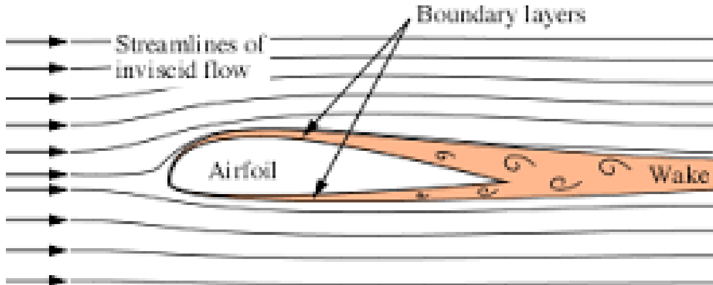
fig. 9 Δημιουργία οριακών στρωμάτων στην επιφάνεια του πτερυγίου.
