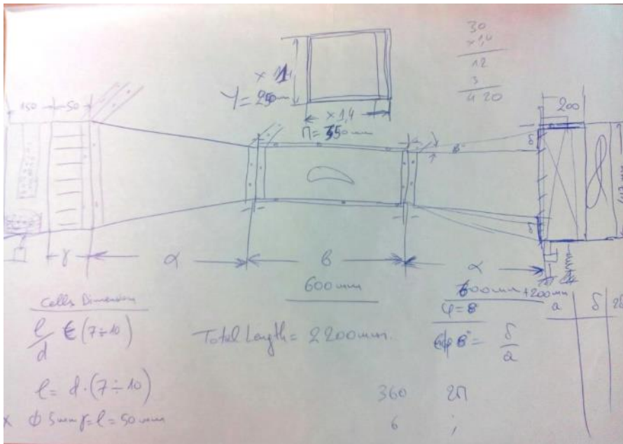
fig. 42 Σκαρίφημα αεροσήραγγας.
