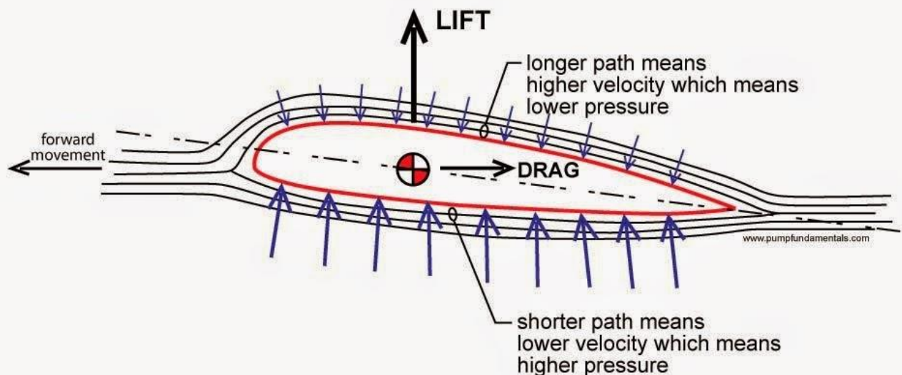
fig. 8 Διαφορά πίεσης σε πτερόγιο.
