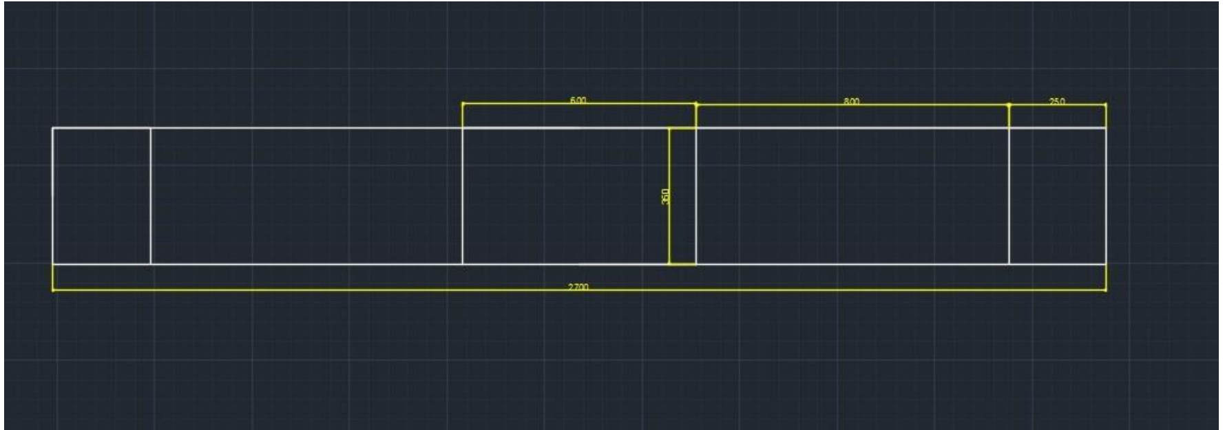
fig. 49 Κάτοψη τελικής γεωμετρίας.
