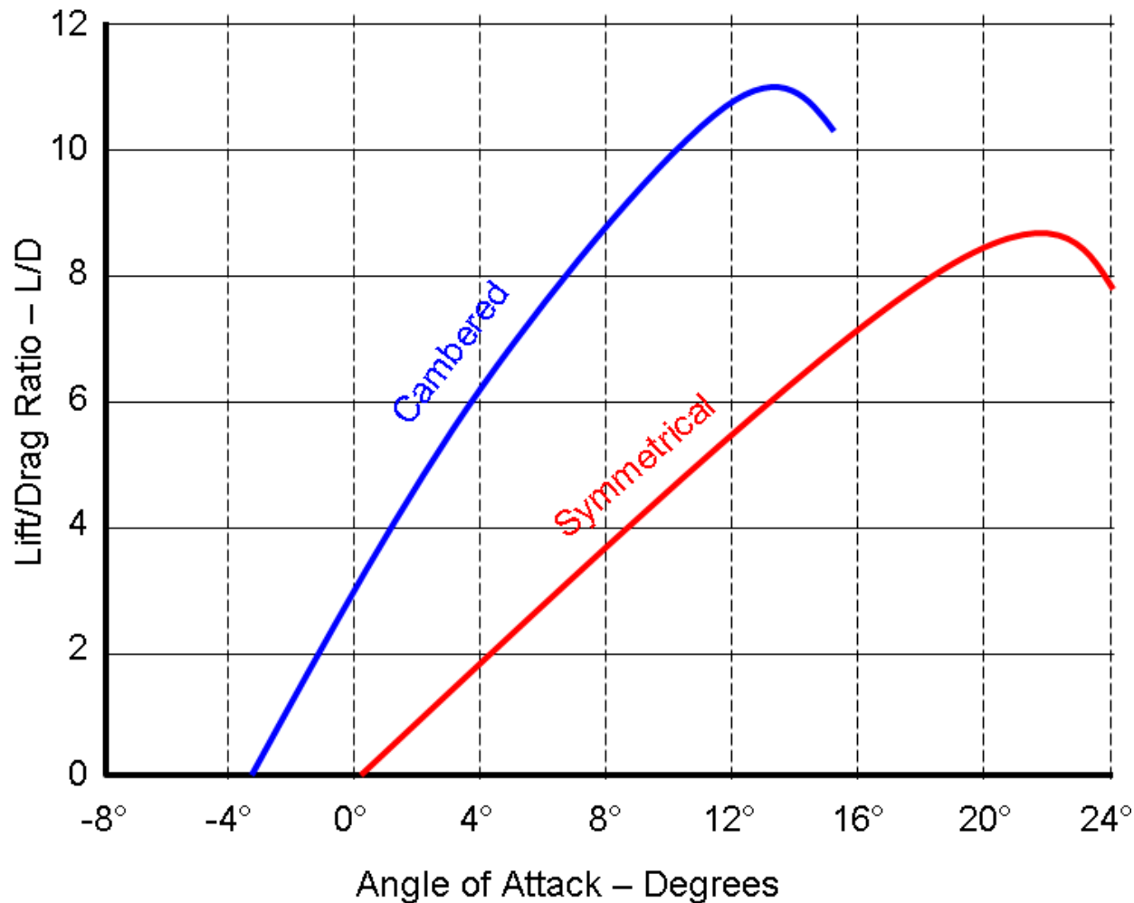
fig. 11 Διάγραμμα αναλογίας άνωσης-οπισθέλκουσας ως προς την γωνία πρόσπτωσης ανέμου για πτερύγιο αεροσκάφους CESSNA T-37 (κυρτό πτερύγιο) και Boeing B-52 Stratofortress (συμμετρικό πτερύγιο).
