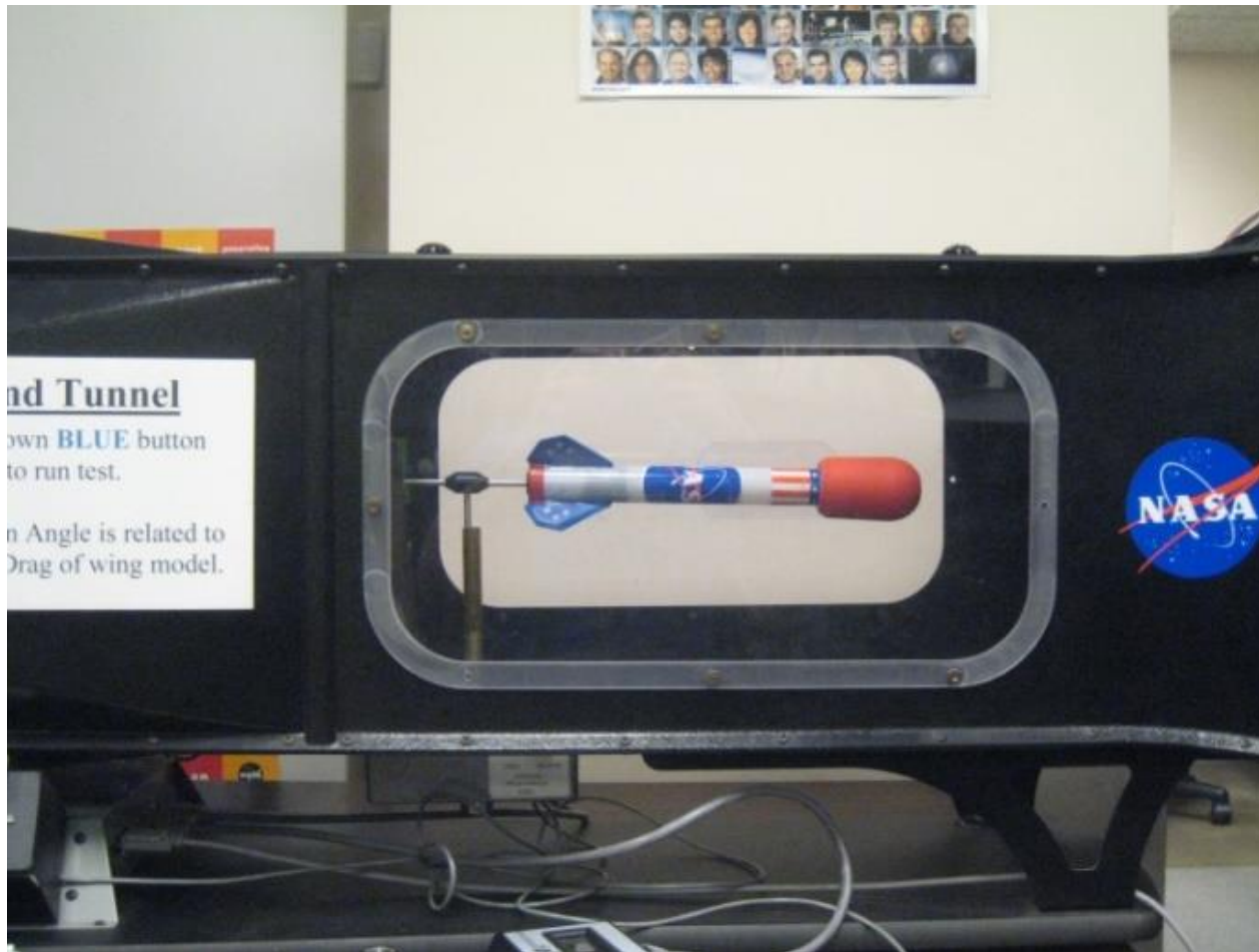
fig. 40 Θάλαμος δοκιμών σε μικρή αεροσήραγγα.
