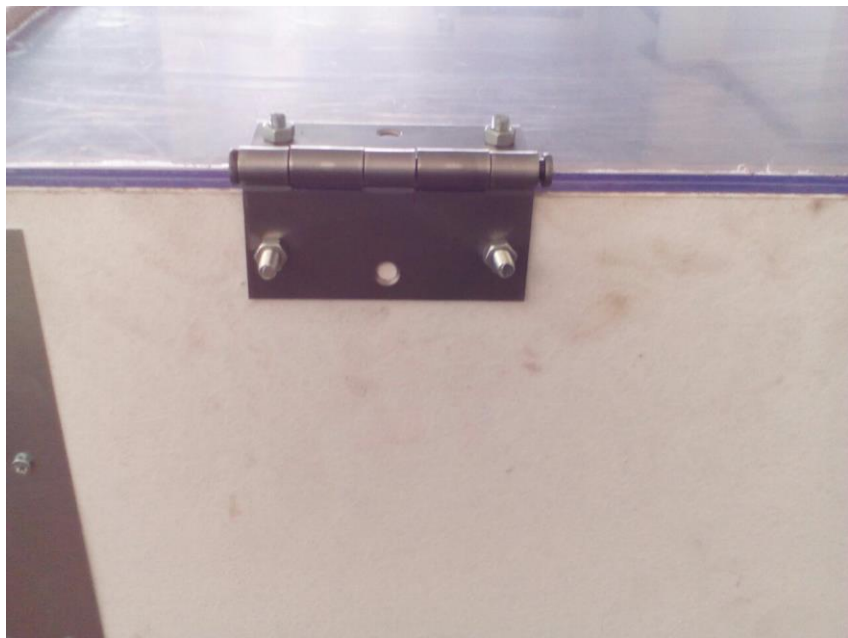
fig. 73 Τοποθέτηση plexiglass με μεντεσέ (Εξωτερική όψη).
