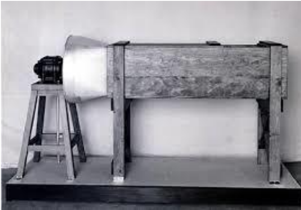
fig. 17 Η αεροσήραγγα των αδελφών Ράιτ.
