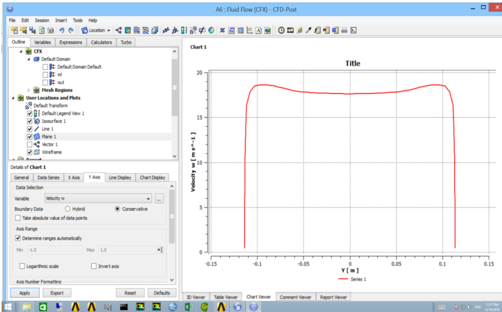
fig. 100 Διάγραμμα σταθερής ταχύτητας στον θάλαμο δοκιμών.
