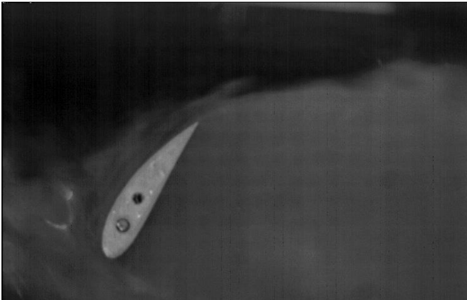
fig. 108 Εικόνα από την βιντεοσκόπηση του πειράματος. Πτερύγιο σε πρόοψη και θέση 55^\circ .
