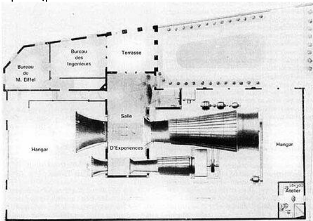
fig. 18 Κάτοψη αεροσήραγγας Eiffel.
