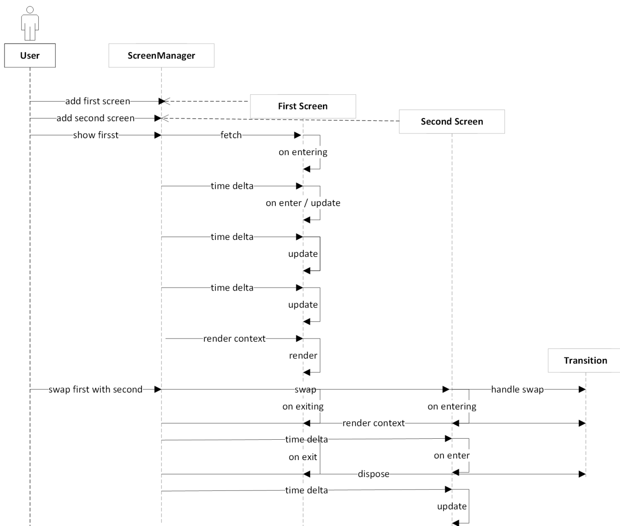
Διάγραμμα 3.3: Διάγραμμα ακολουθίας του υποσυστήματος διαχείρισης οθονών
