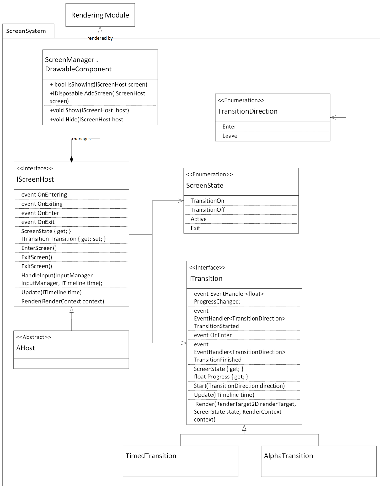
Διάγραμμα 3.4: UML του υποσυστήματος διαχείρισης οθονών
