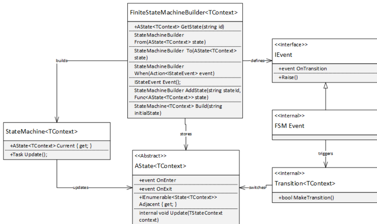
Διάγραμμα 3.13: UML του υποσυστήματος των state machines
