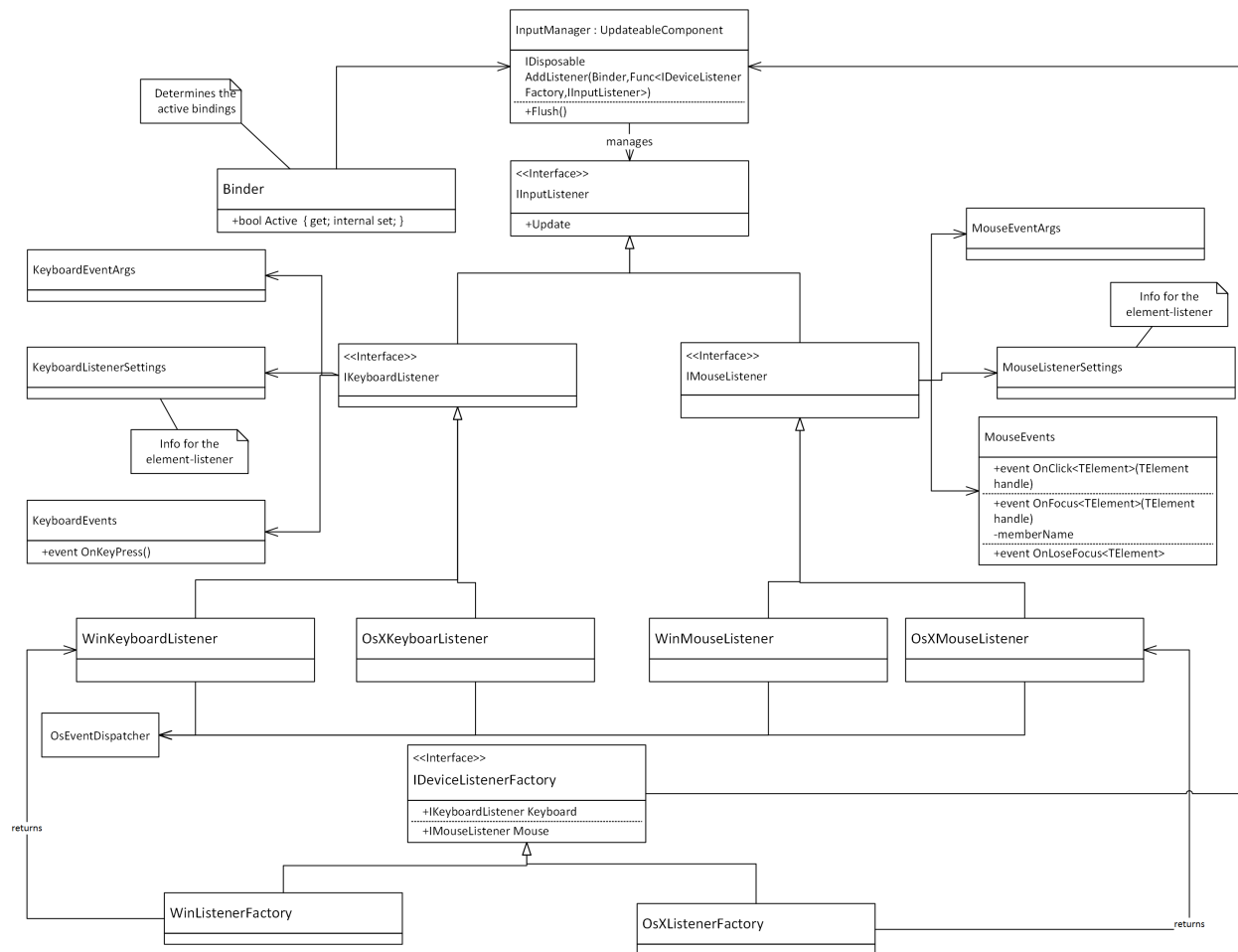
Διάγραμμα 3.5: Αρχιτεκτονική υποσυστήματος διαχείρισης εισόδων
