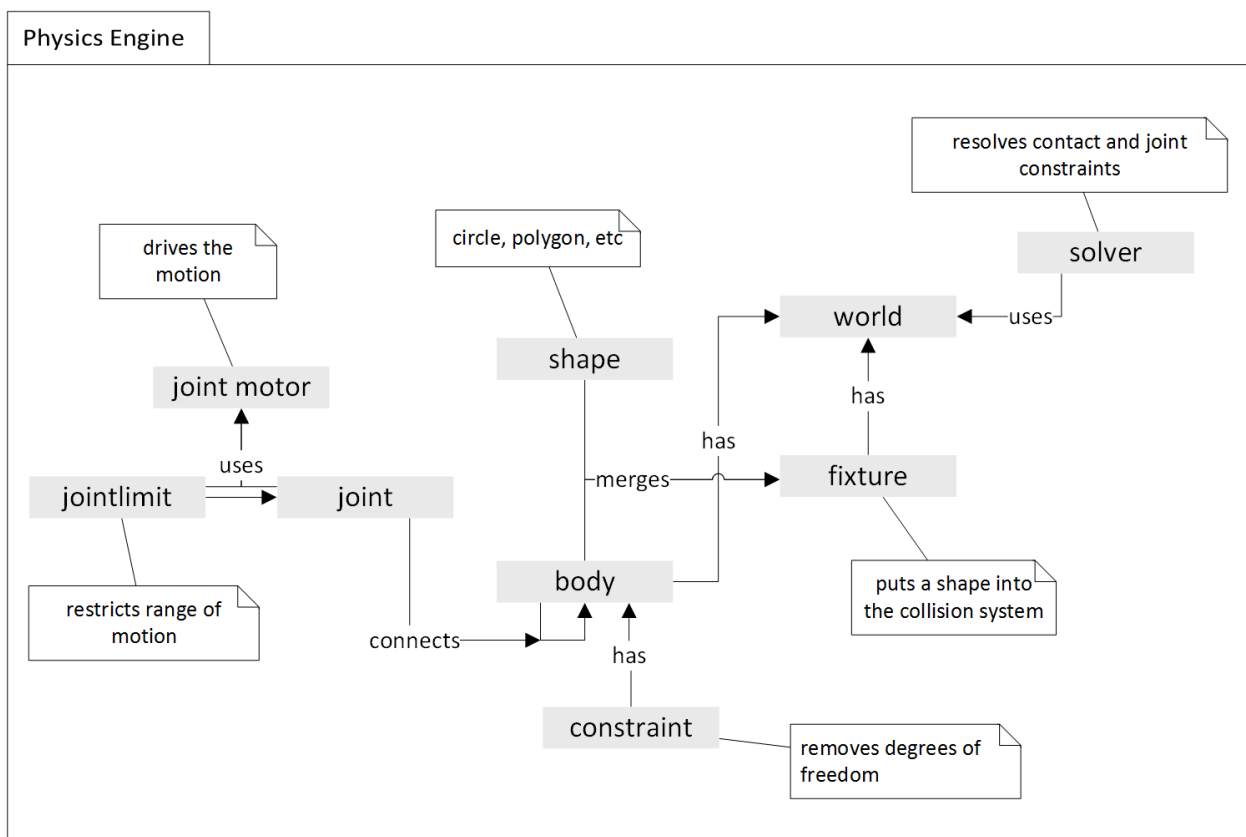
Διάγραμμα 3.6: Υποσύστημα φυσικής και εντοπισμού συγκρούσεων
