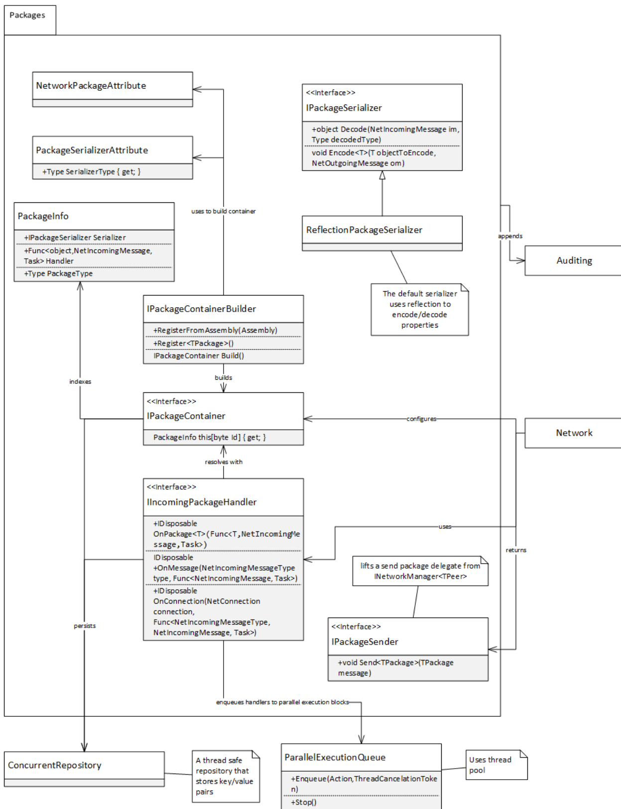
Διάγραμμα 4.3: Υποσύστημα διαχείρισης πακέτων
