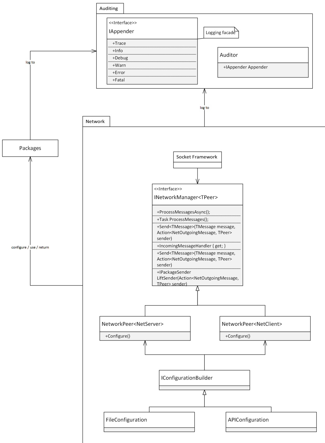
Διάγραμμα 4.4: Μονάδα διαχείρισης της δικτύωσης
